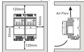
Установка вплотную (-10 ... +40°C)
